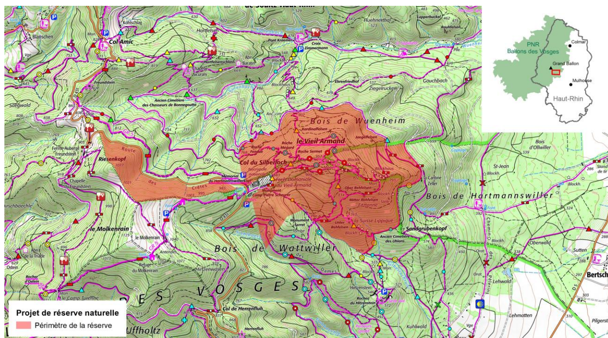
▲ Figure 1. Plan de situation du projet de réserve naturelle du Hartmannswillerkopf – Vieil-Armand.
