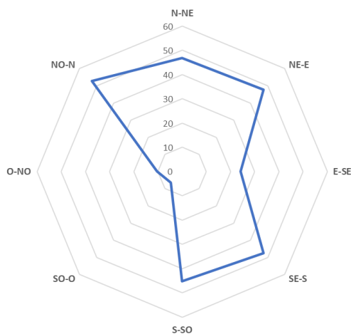
▲ Figure 10. Surfaces par type d'exposition.
