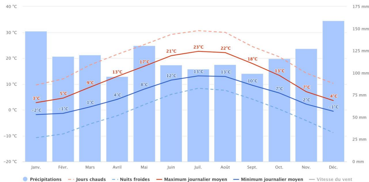
▲ Figure 6. Températures et précipitations moyennes modélisées au sommet du Hartmannswillerkopf (956 m). Source : Météoblue.
