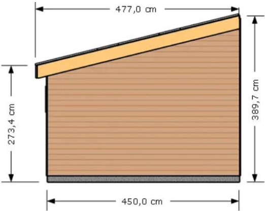
Façade EST
