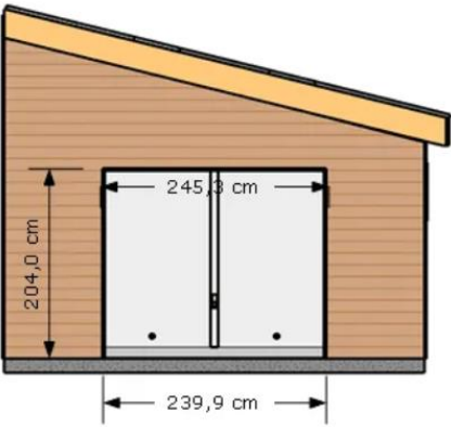
Façade OUEST
