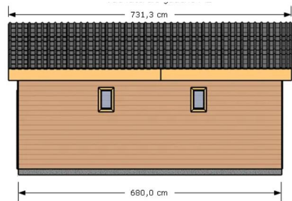
Façade SUD
